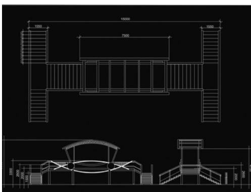
Переходной пешеходный мост через магистральные трубы. Он же может использоваться как пешеходный мост через канал
