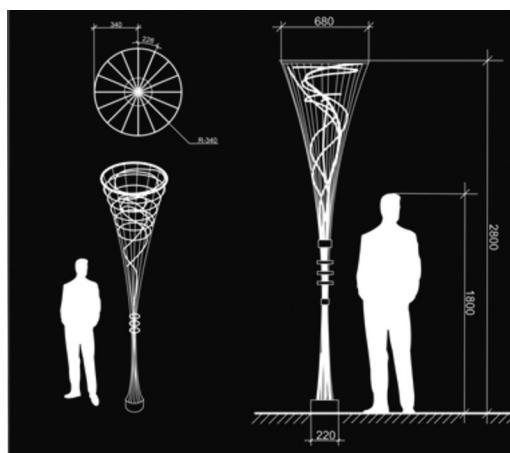
Уличный фонарь на неоновых лампах
